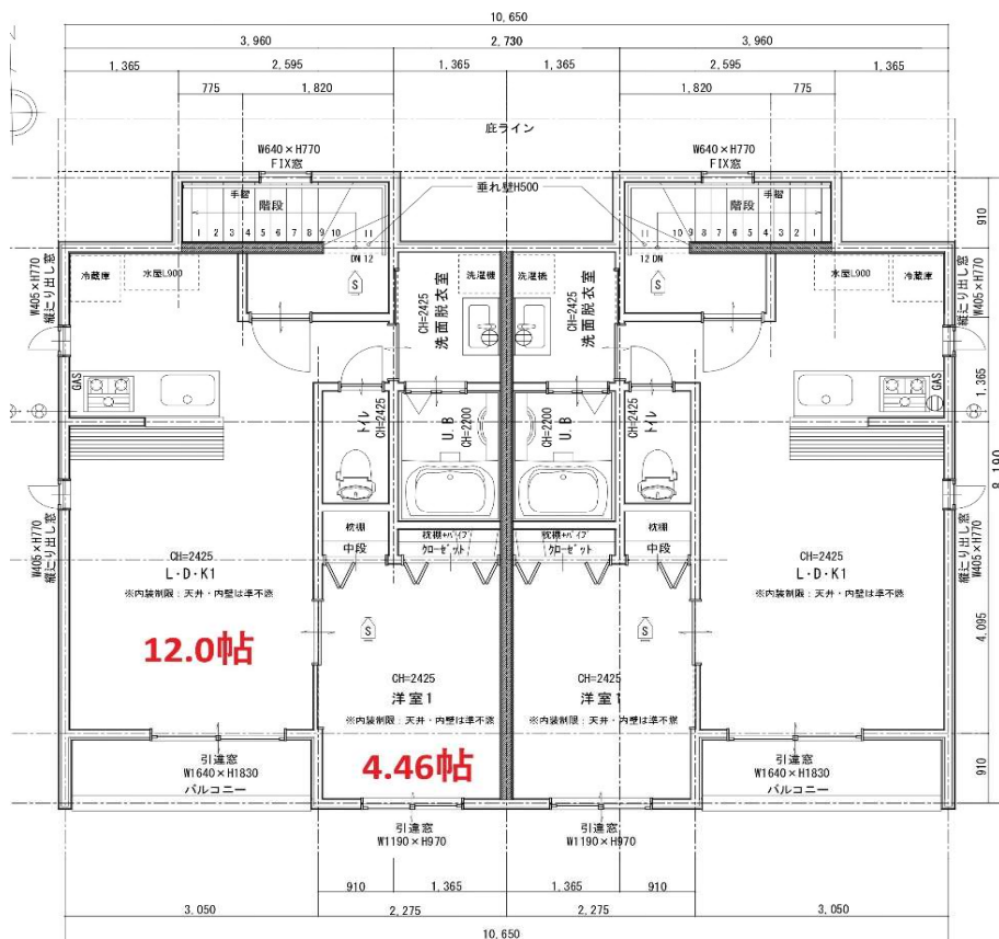
2階平面図 S=1/60
