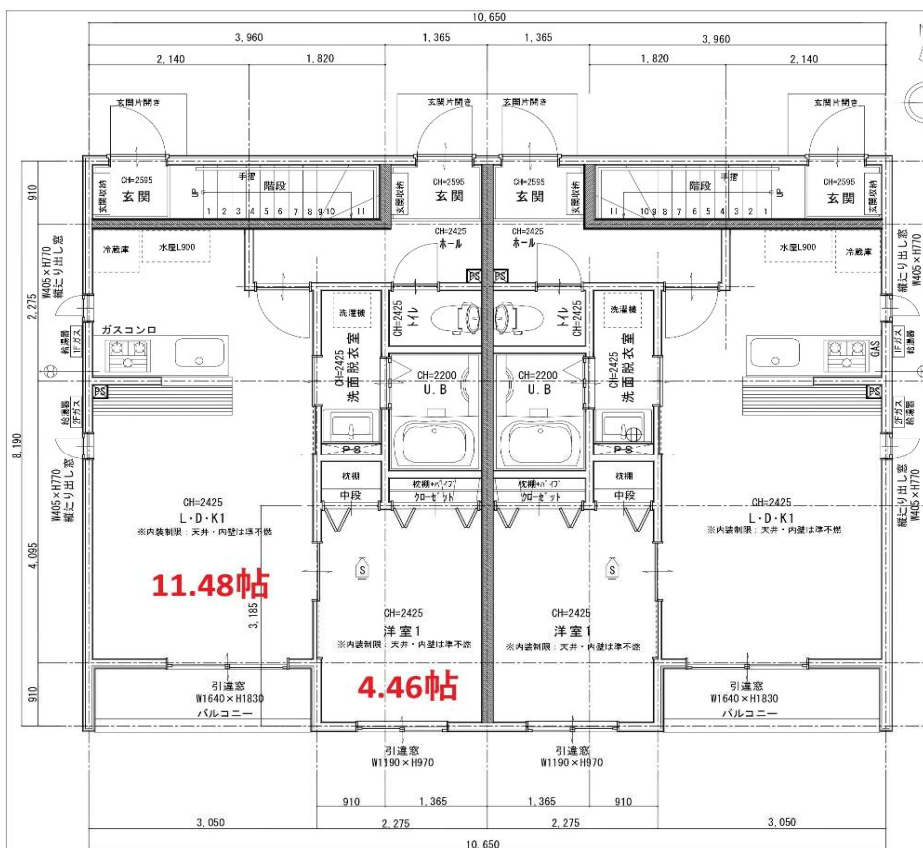
1階平面図 S=1/60
