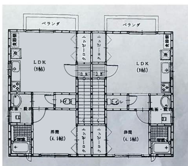
2階 平面図
