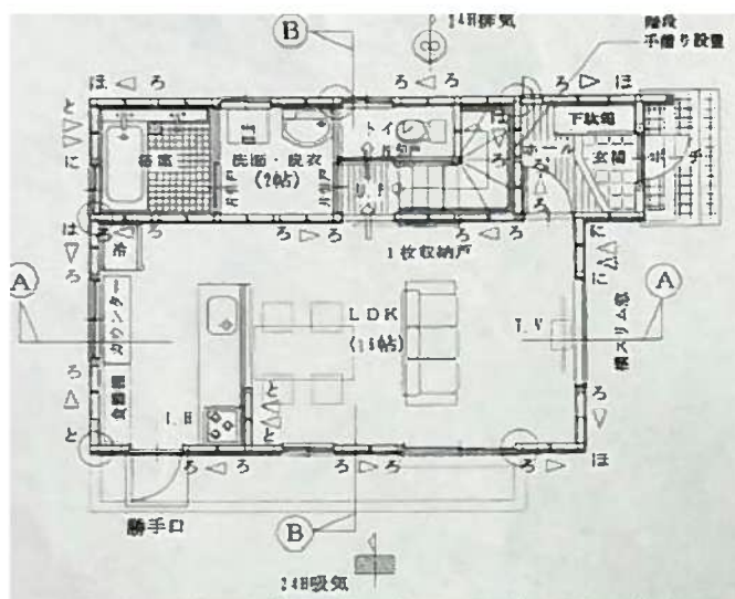
1階 平面図
