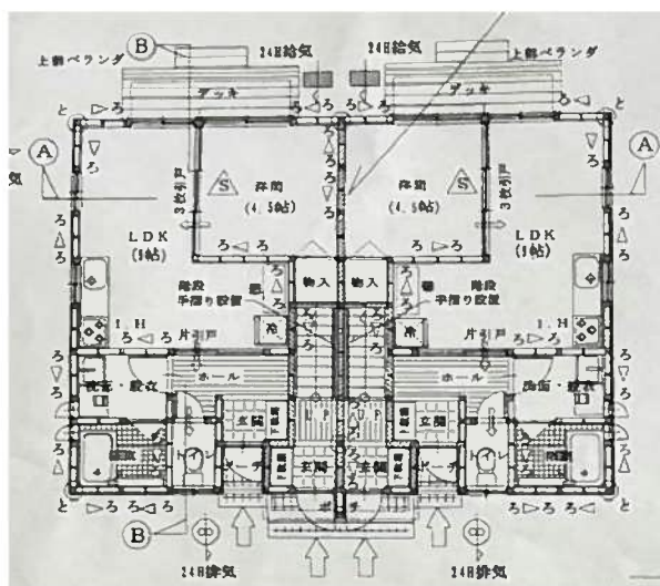
1階 平面図
