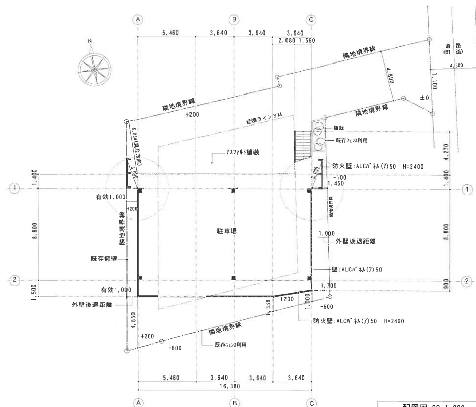
配置図 SC 1:200
